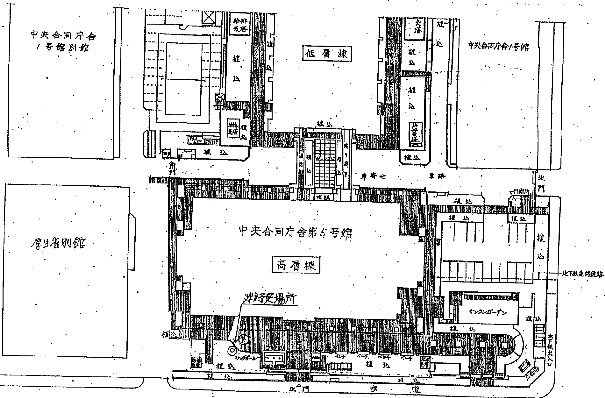
中央合同庁舎第5号館配置図
